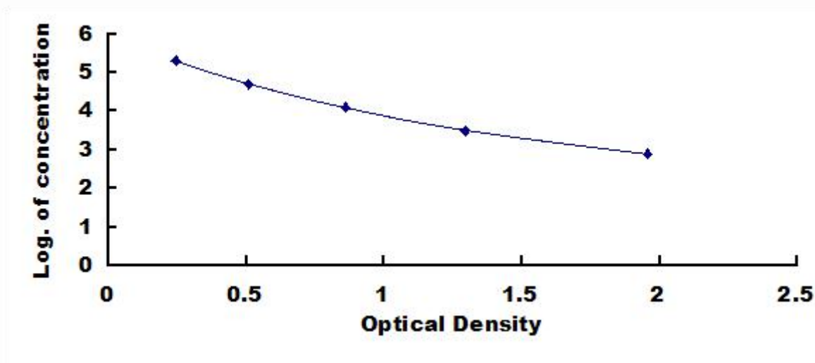
叶酸(FA)检测试剂盒标准曲线
